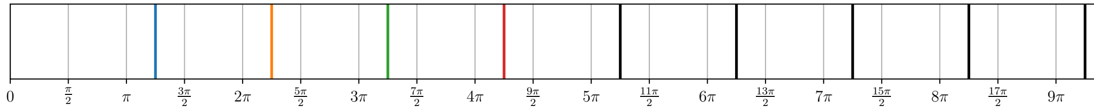
Eigenwerte \kappa_n l
