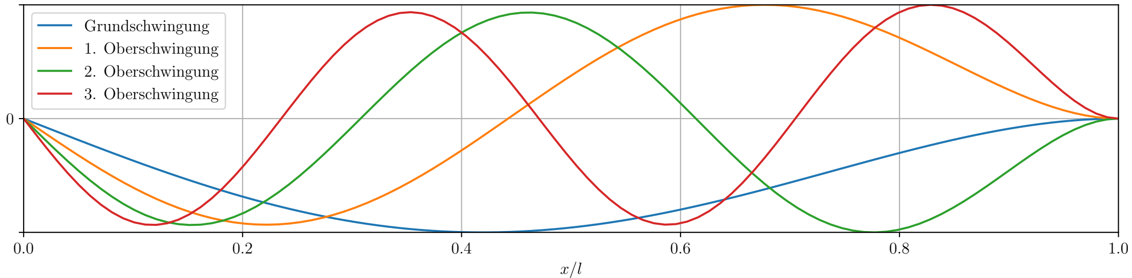
Eigenformen W_n(x)
