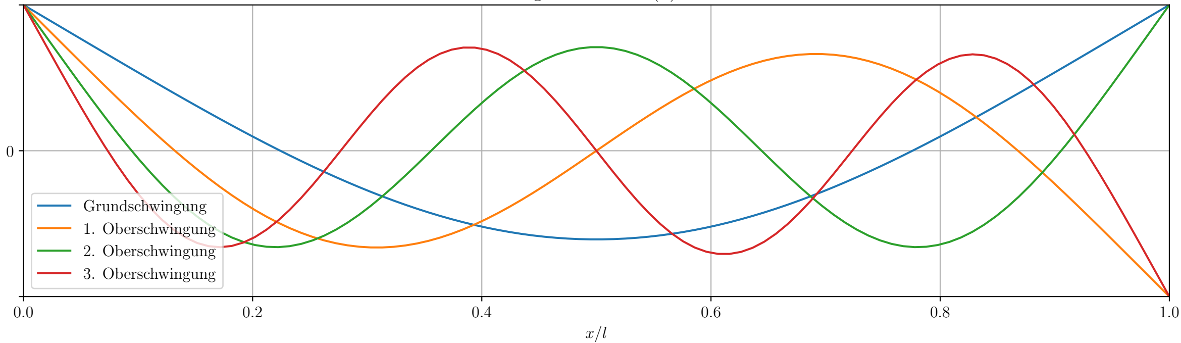
Eigenformen W_n(x)
