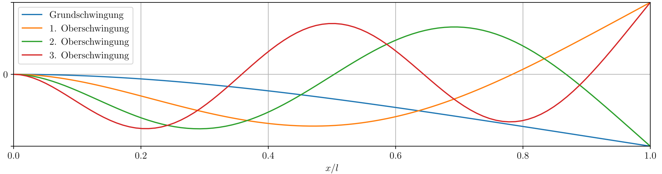
Eigenformen W_n(x)
