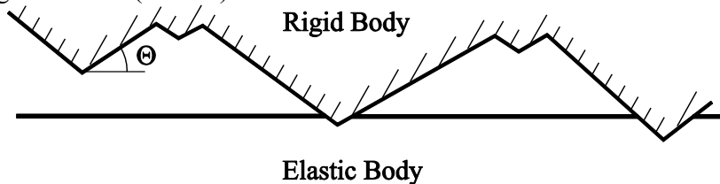
Abb. 3 Kontakt zwischen einer rauen Fläche bestehend aus kegelförmigen Spitzen und einem elastischen Körper.
