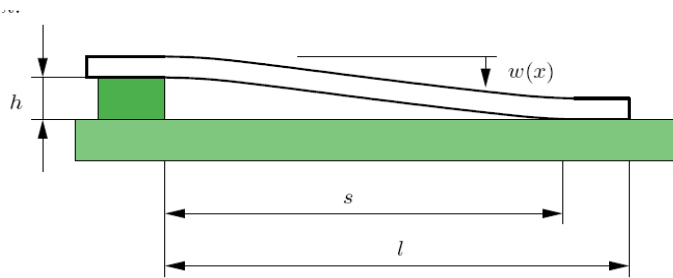
Abb. 1 Adhäsiver Kontakt eines mikromechanischen Modells
