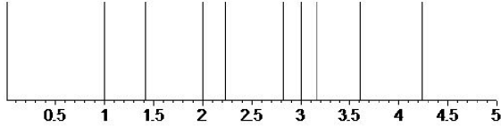
Bild 1. Verteilung von Eigenfrequenzen einer Membran bei a = b .
